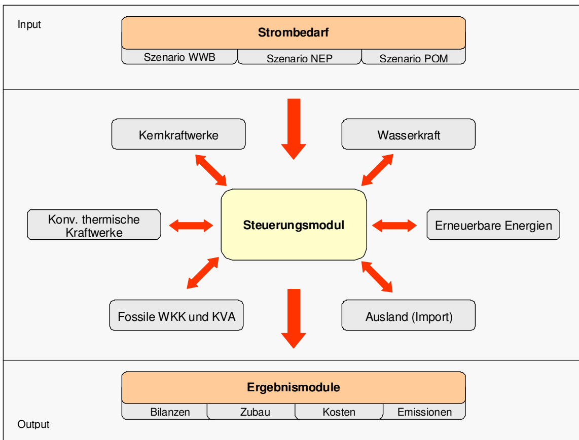
Figur 2-8: Modellaufbau
