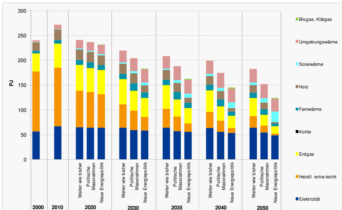
Figur 5-27: Szenarienvergleich Private Haushalte Endenergienachfrage nach Energieträgern 2000 – 2050, in PJ
