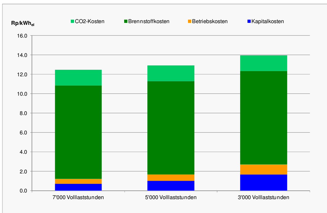
Figur 6-3: Gesamtwirtschaftliche Stromgestehungskosten von neuen Gaskombikraftwerken in der Schweiz (Bezugsjahr 2030, Szenario „Weiter wie bisher“), in Rp/kWh el
