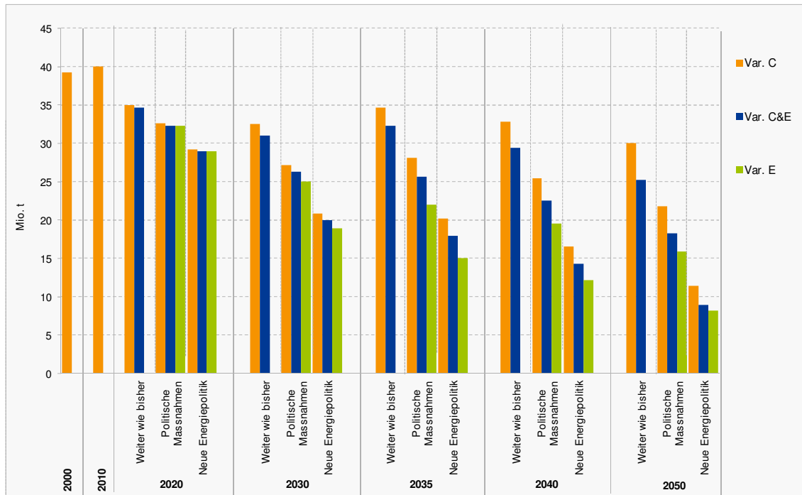
Figur 5-20: Szenarienvergleich CO 2 -Emissionen* nach Szenarien und Varianten, in Mio. t
