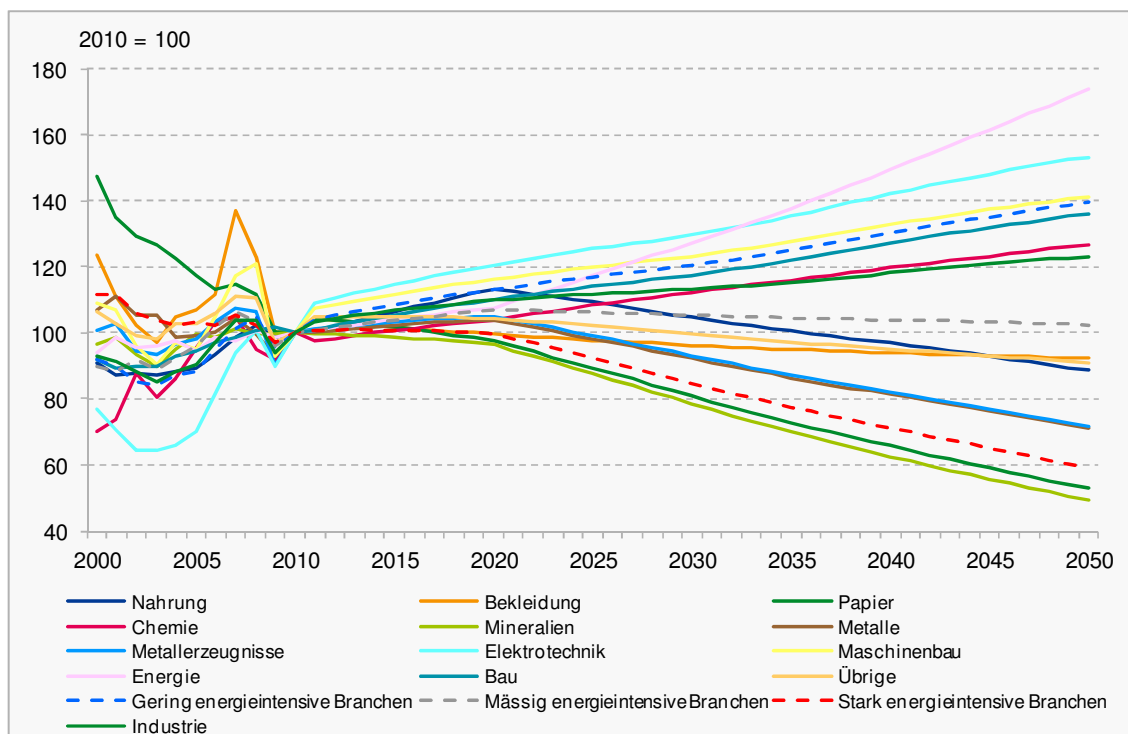
Figur 7-17: Szenario „Weiter wie bisher“, Industriesektor Produktionsmenge nach Branchen 2000 – 2050, indiziert (2010 = 100)
