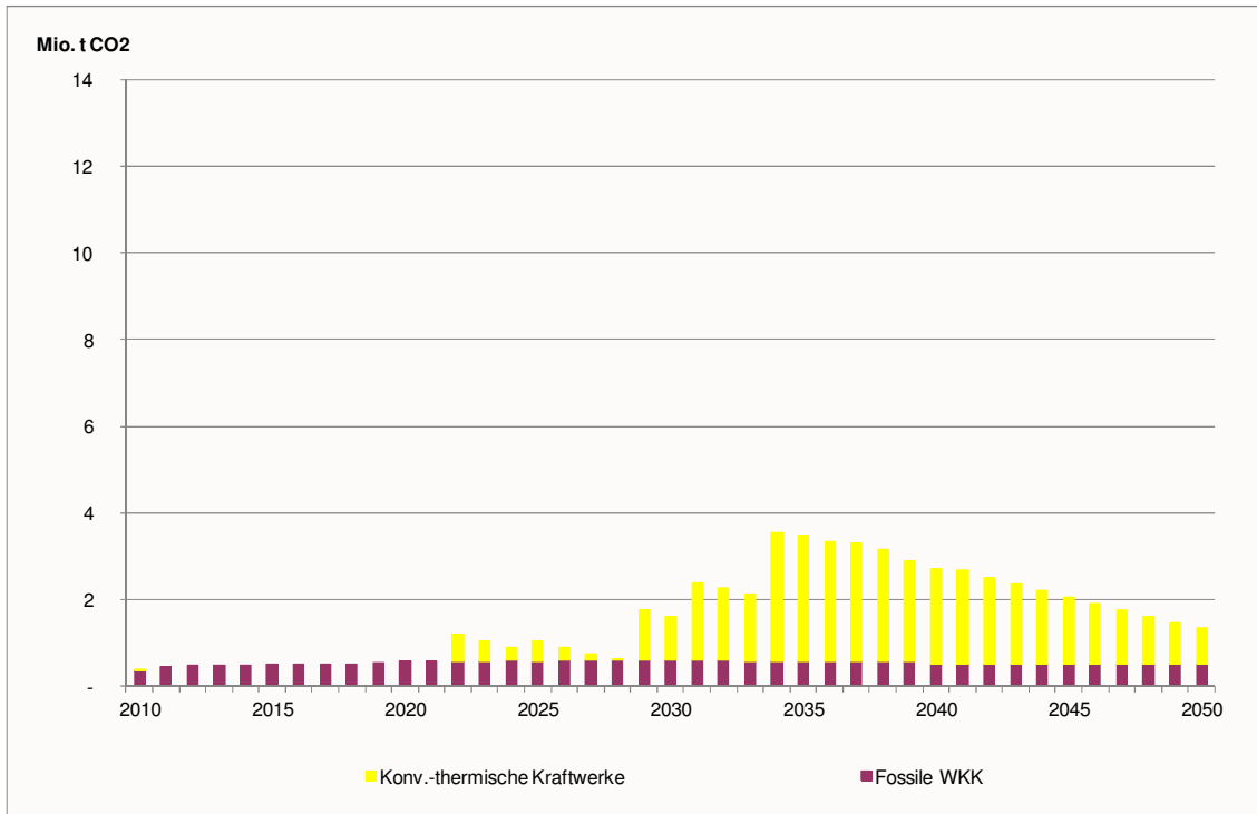
Figur 8-60: Szenario „Neue Energiepolitik“, Variante C&E CO 2 -Emissionen inkl. Wärmegutschriften, hydrologisches Jahr, in Mio. t CO 2 /a
