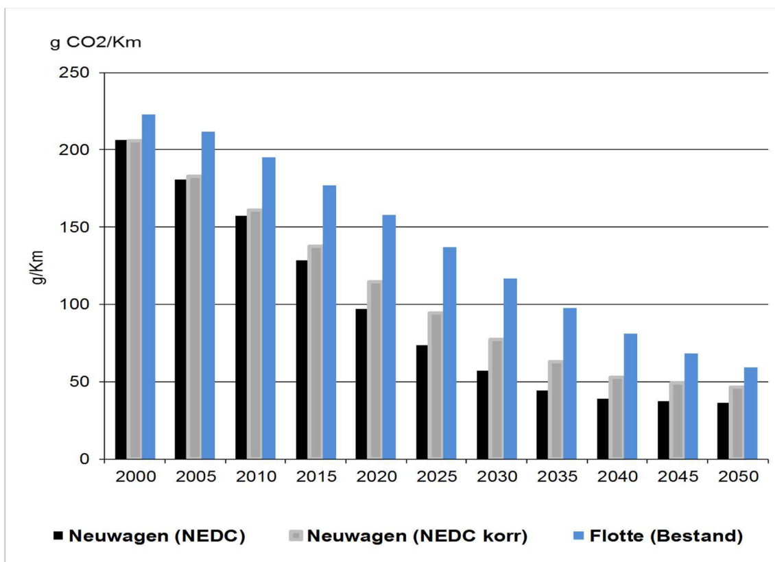
Figur 8-23: Szenario „Neue Energiepolitik“, Verkehrssektor Entwicklung der mittleren CO 2 -Emission der Neu-PW bzw. der PW-Flotte 2000 - 2050 (in g CO 2 /km)
