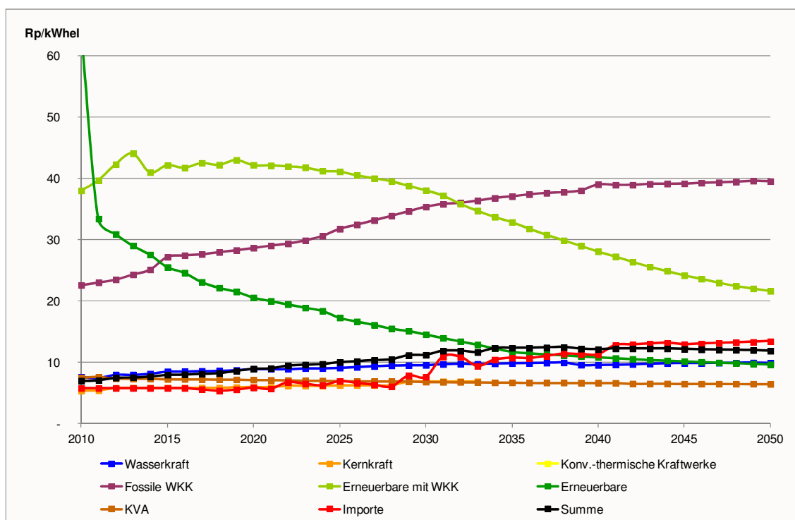
Figur 8-67: Szenario „Neue Energiepolitik“, Variante E Gestehungskosten des Kraftwerksparks, in Rp/kWh el
