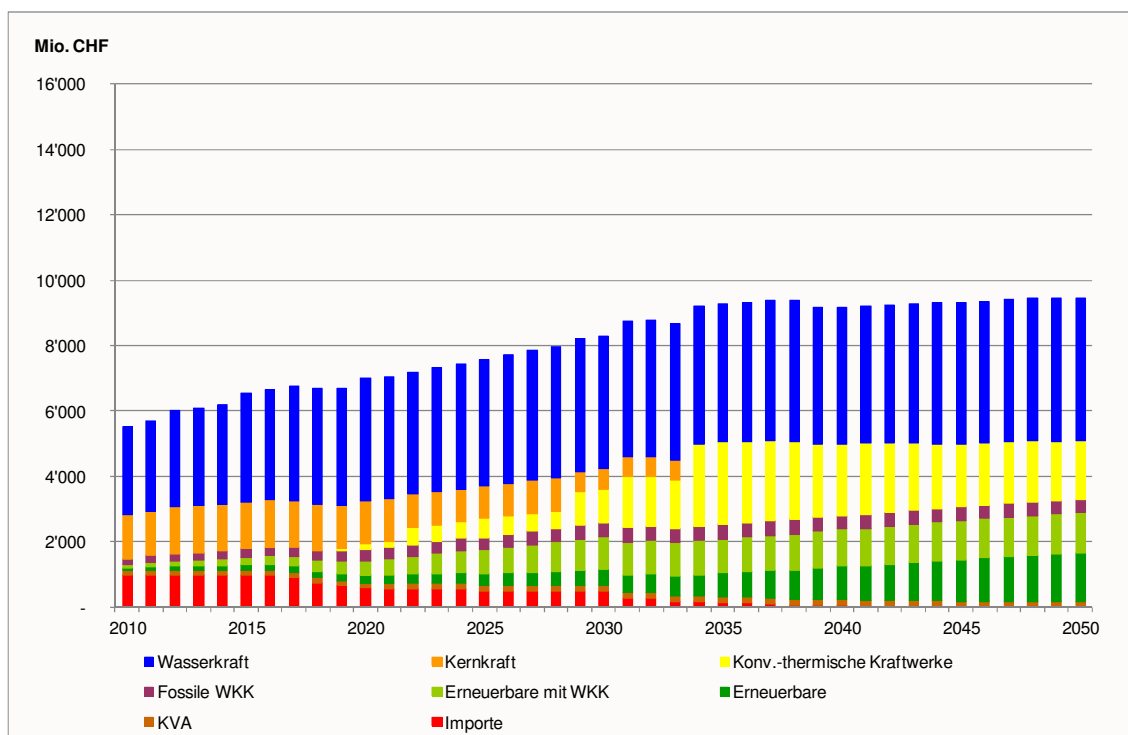
Figur 7-66: Szenario „Weiter wie bisher“, Variante C&E Jahreskosten des Kraftwerkparcs, in Mio. CHF/a
