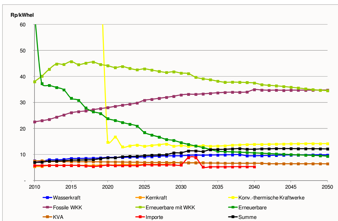
Figur 9-58: Szenario „Politische Massnahmen“, Variante C Gestehungskosten des Kraftwerksparks, in Rp/kWh el
