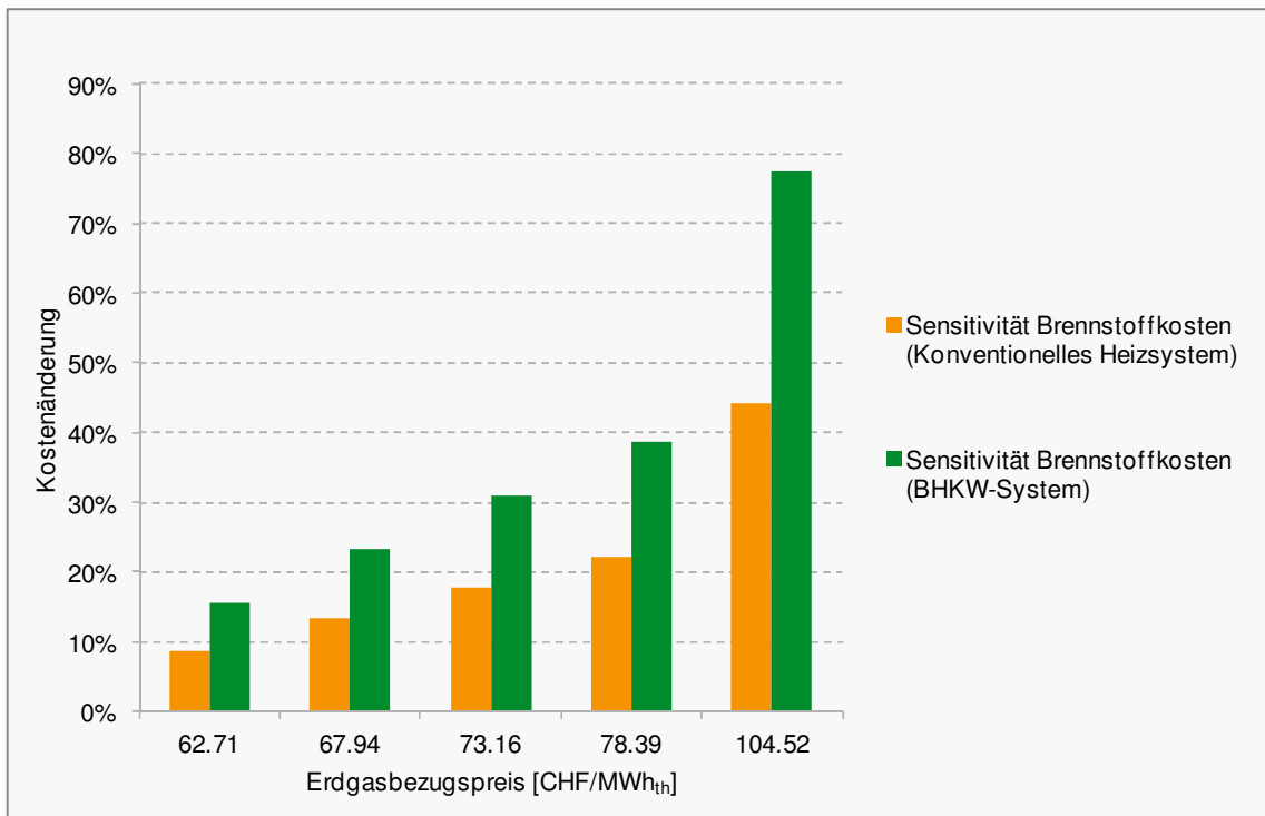
Figur II.2-23: Gegenüberstellung eines konventionellen Heizsystems und eines BHKW-Systems (Kategorie 3, 1'000 kW el ) hinsichtlich der Sensitivität auf des Erdgasbezugspreis auf die Jahreskosten im Jahr 2010
